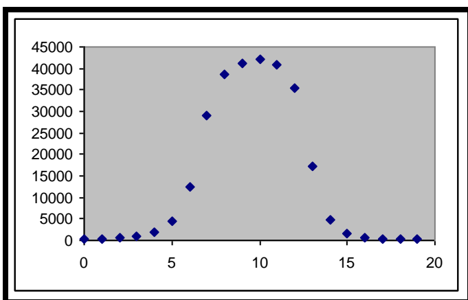
Fig.2. Perfil de una estrella no saturada (gaussiana)
