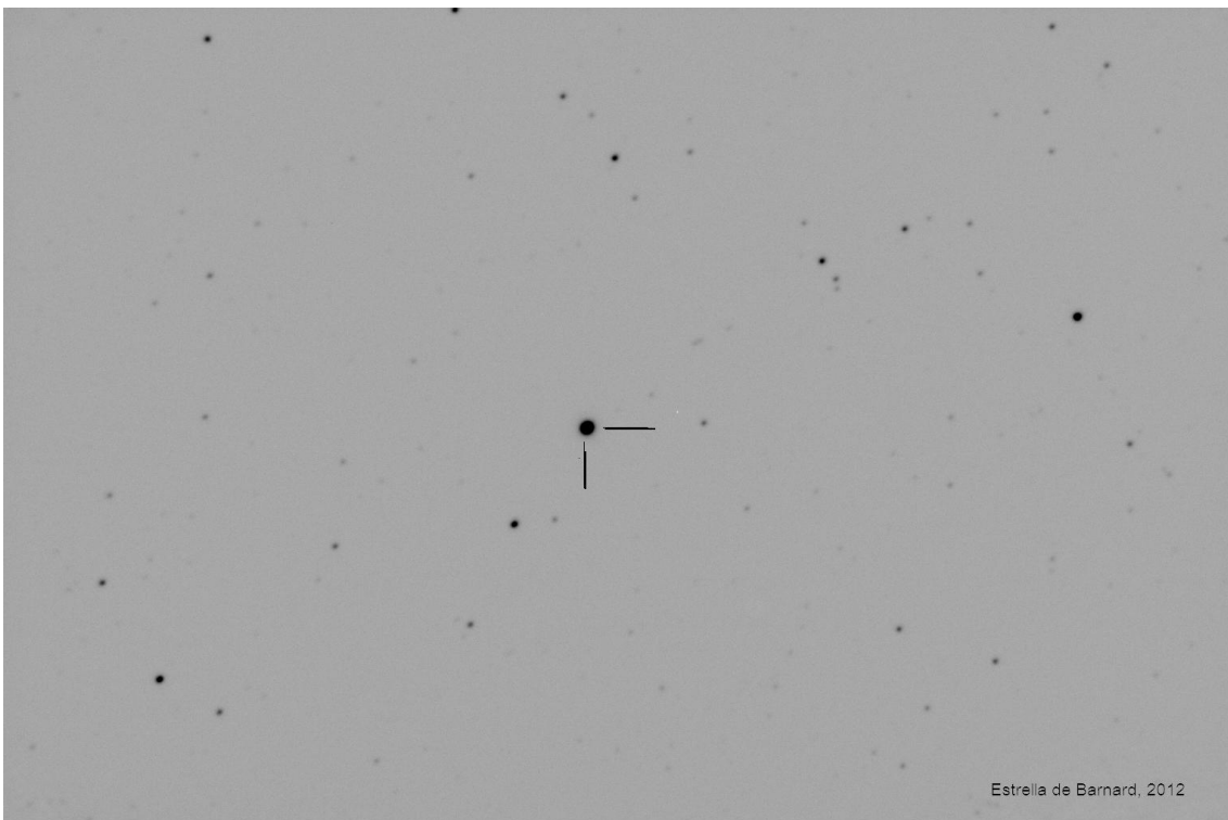
Fig.1b- Campo estelar con la estrella de Barnard (retículo) en el año 2004
