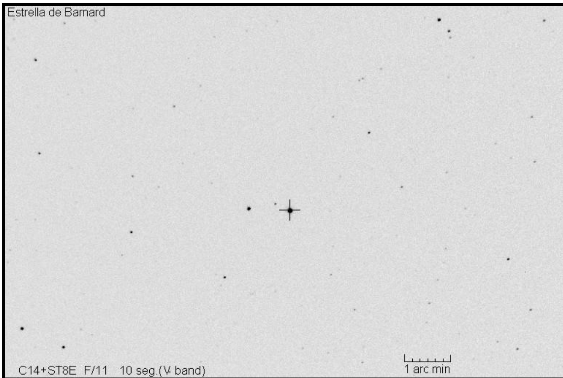
Fig.1a- Campo estelar con la estrella de Barnard (cruz) en el año 2004
