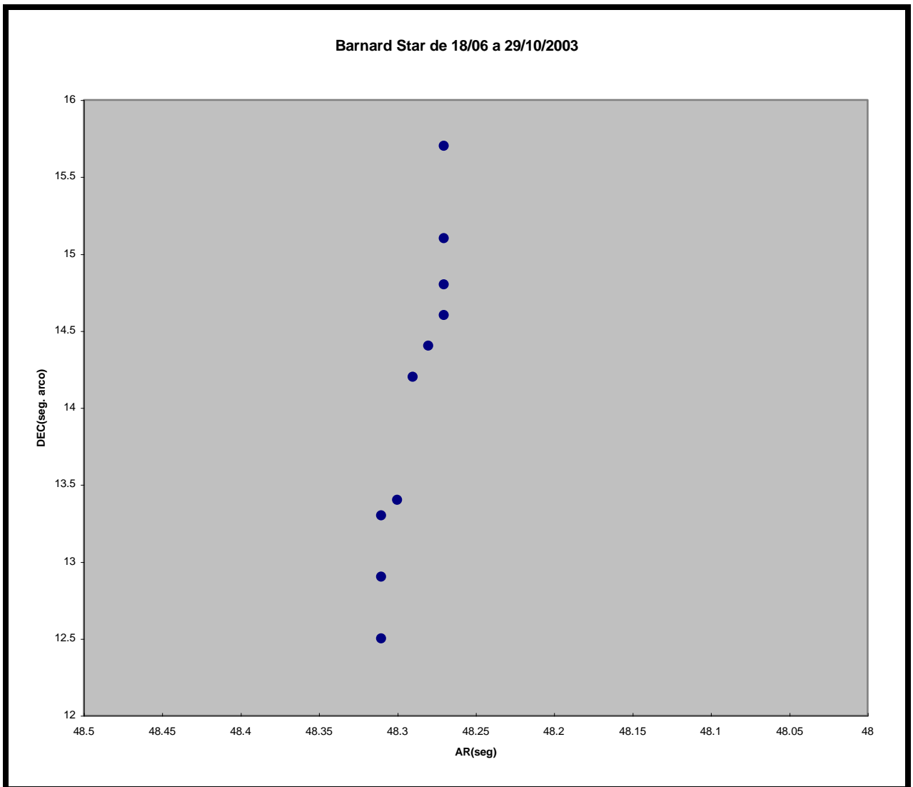
Fig. 6. Puede verse en el gráfico que el movimiento propio de la estrella y una pequeña modulación lateral
